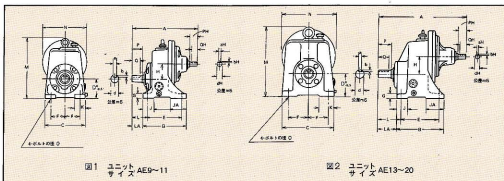
寸法表
