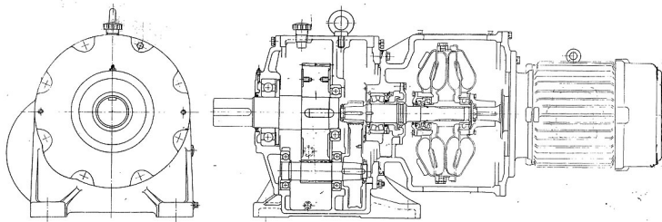
30EFB-H21 (4-30) 内部構造図
