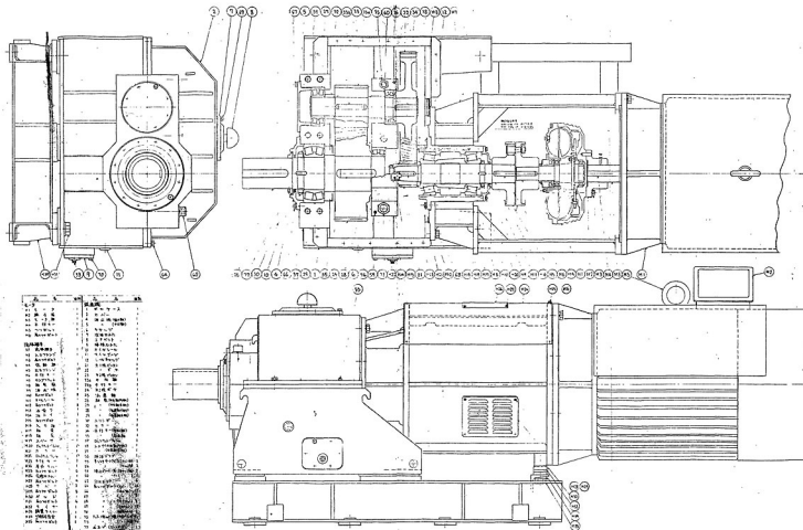
30EF-H36 (6-90) 内部構造図
